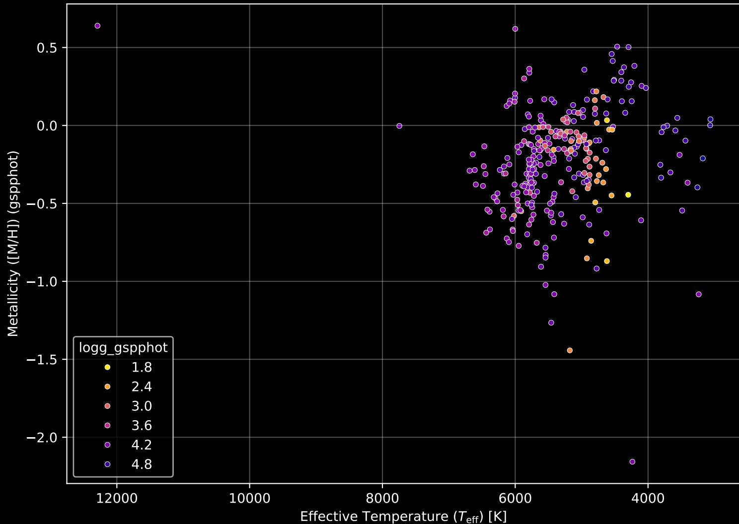
APOGEE DR17 Field: [178-48_MGA] Stellar Population Parameters (n= 303)
